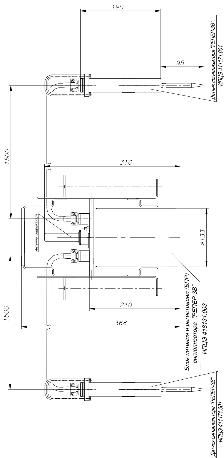
Рисунок 3. Сигнализатор прохождения очистного устройства "РЕПЕР-3В" Габаритный чертеж
